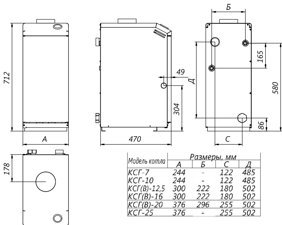
Рисунок 1 - Общий вид, габаритные и присоединительные размеры котлов модели «КСГ(В)»
